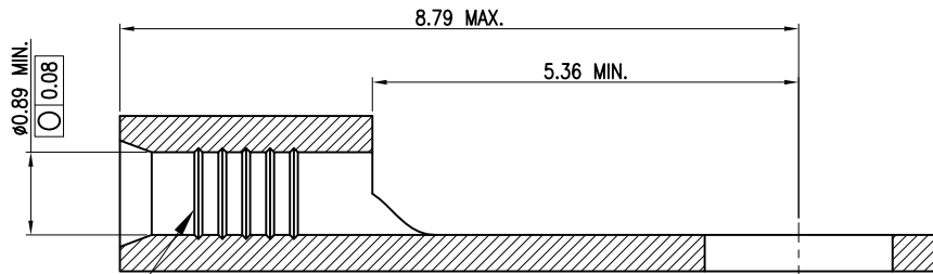
SECTION A-A
